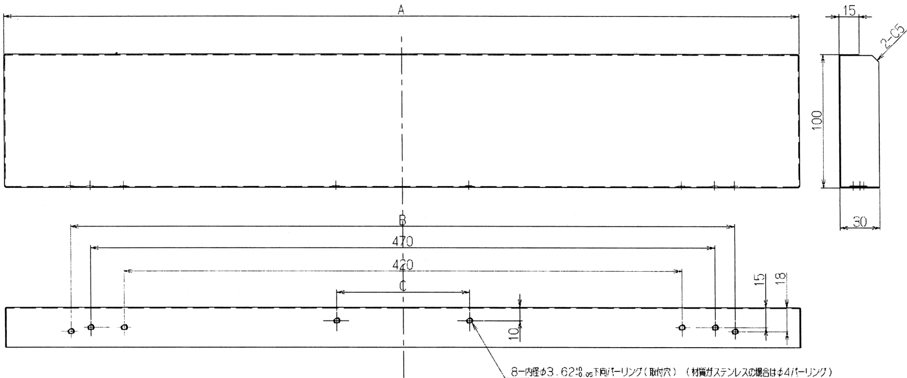
8-内径φ3.62mm 0.05 下向バーリング(取付穴) (材質がステンレスの場合はφ4バーリング)
